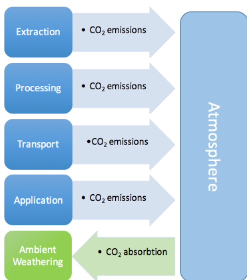
Figuur 2. Opzet voor de eigen berekening van de ketenemissies (optie b uit Methodedocument, paragraaf 4)
